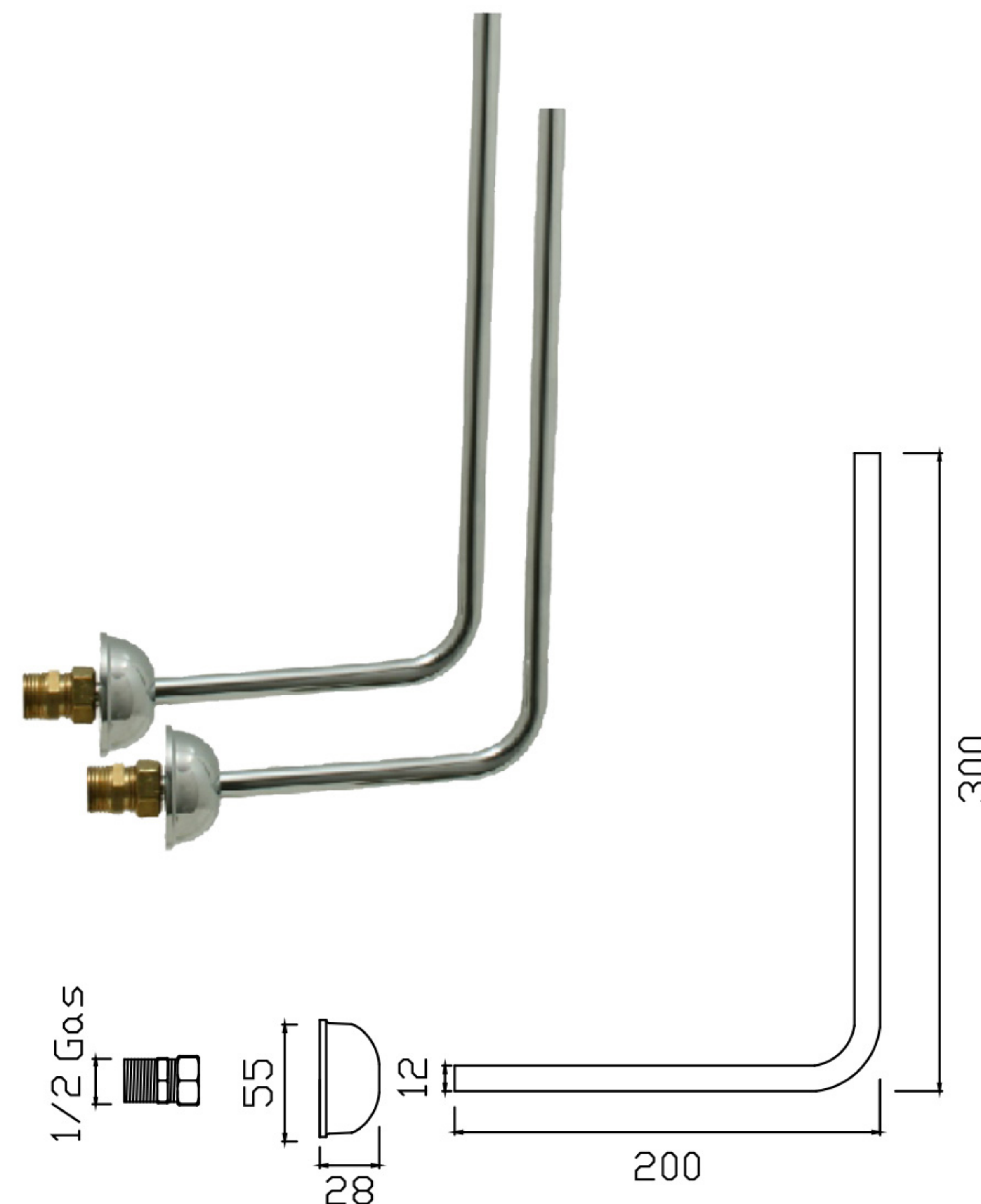
ART 255 Coppia curvette sottolavabo per batteria 3 fori
