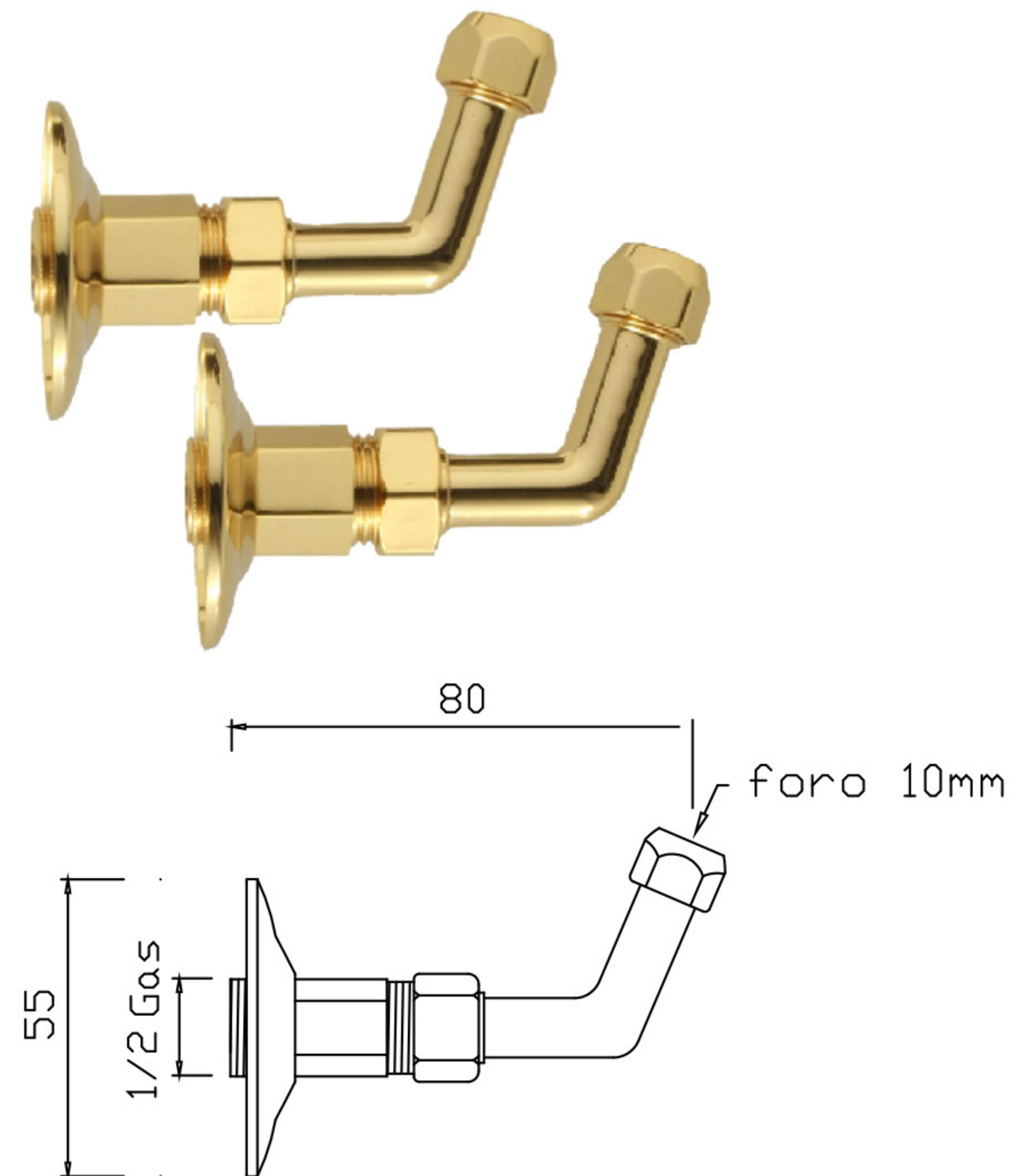
ART 256 Coppia di raccordi curvi per monoforo
