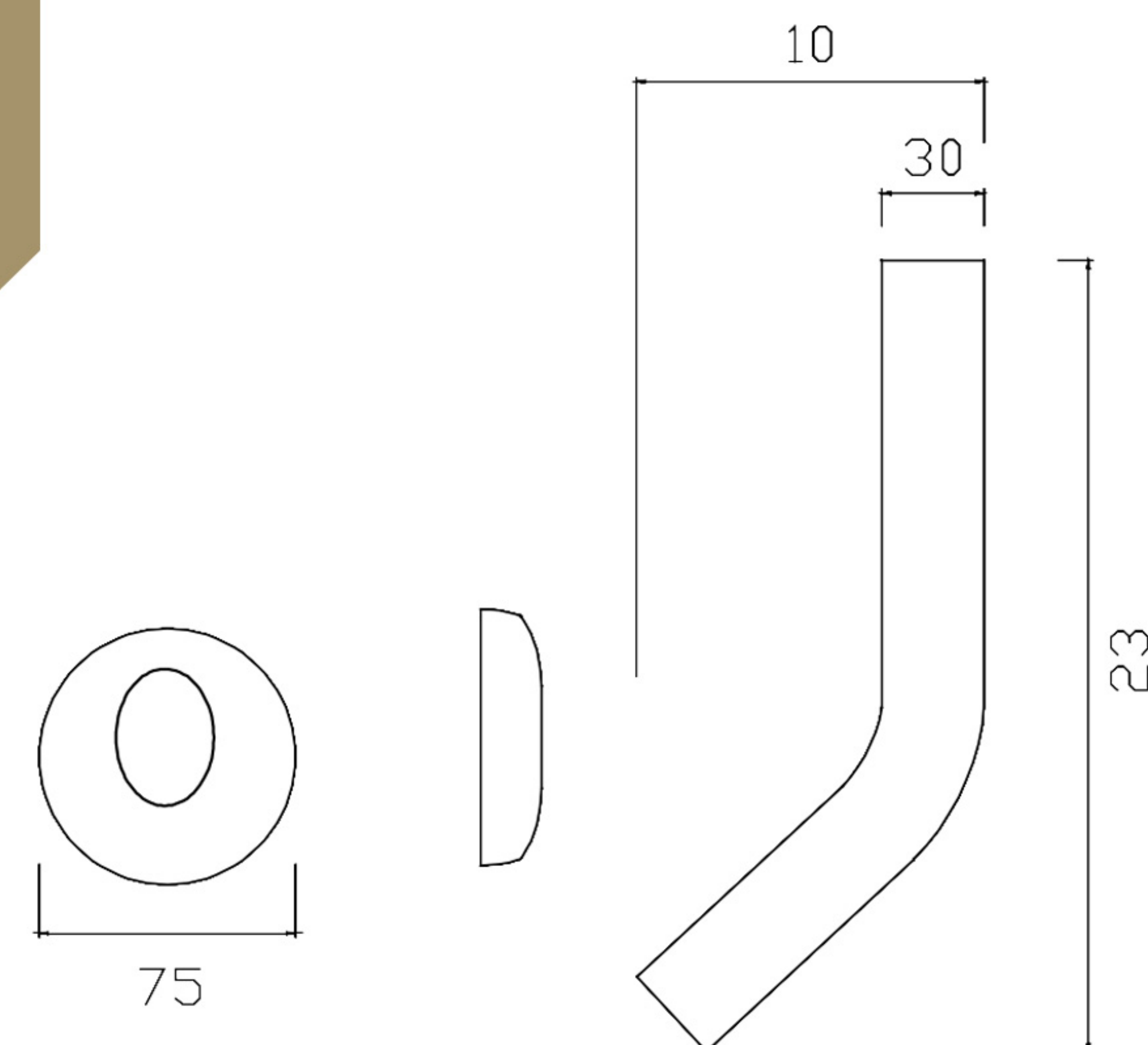
ART 204 Tubo cartellato L= 300mm
