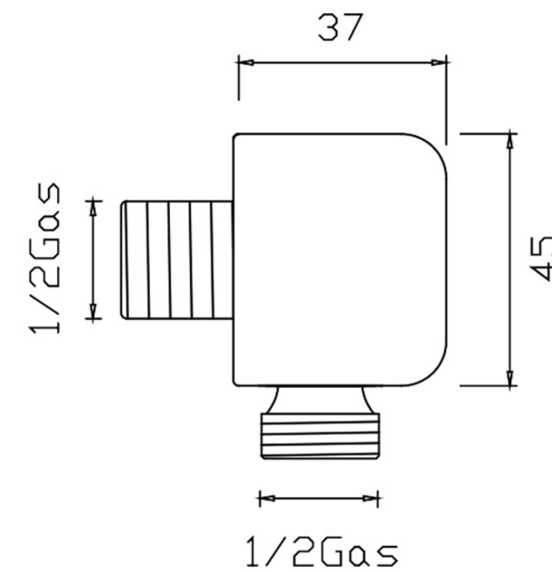
ART 181 Presa acqua da parete
